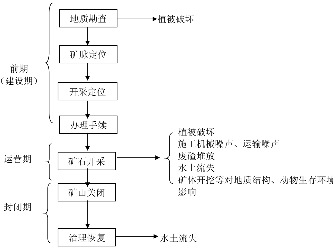
图3-1 矿山开采工艺流程及污染流程
