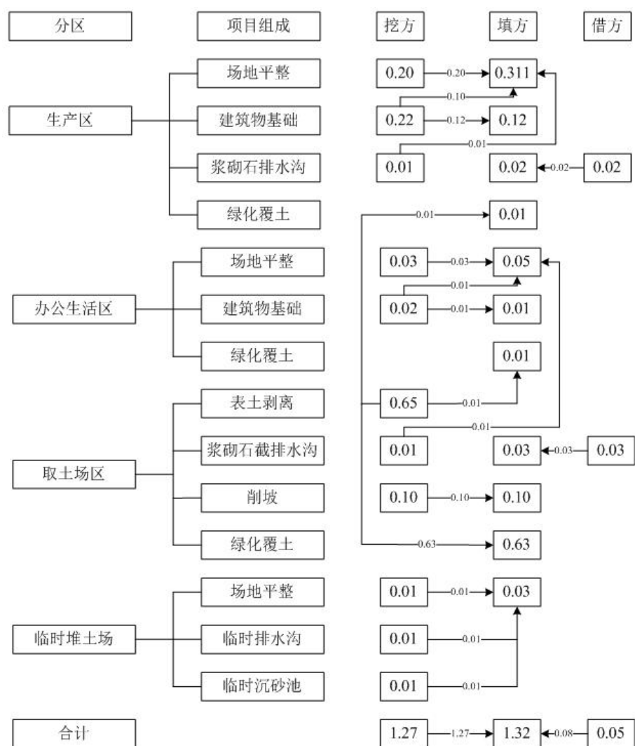
图3-6 本项目土石方平衡示意图单位：万m³
