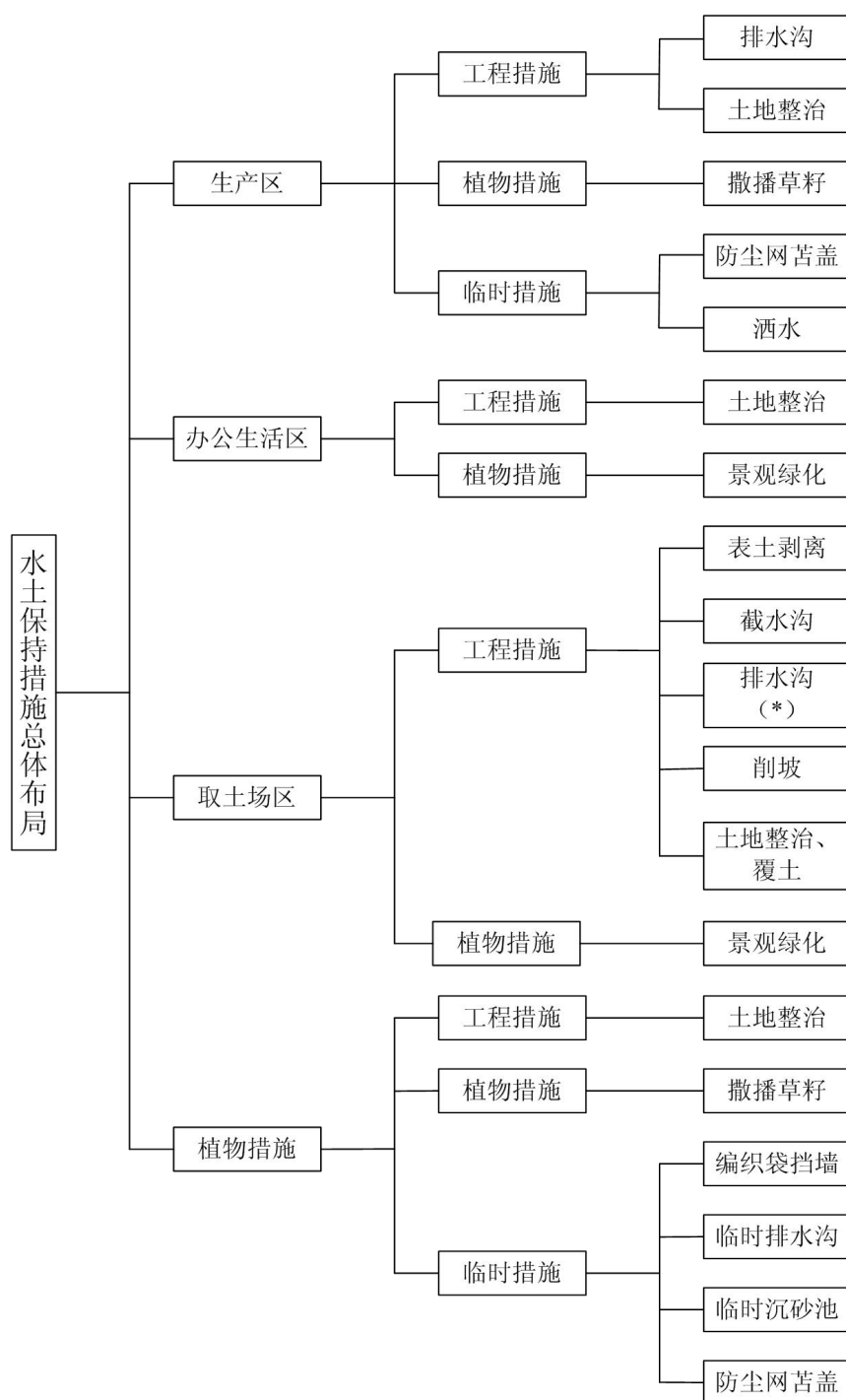
图6-1 水土流失防治措施体系框图
