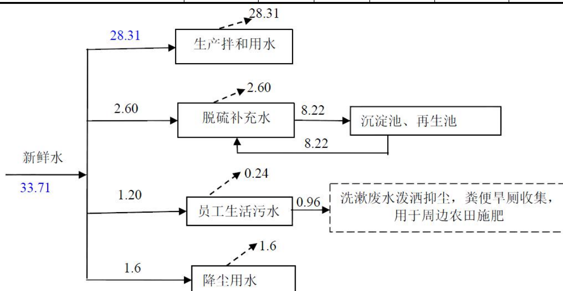
图 2-7 项目水平衡图单位：m 3 /d
