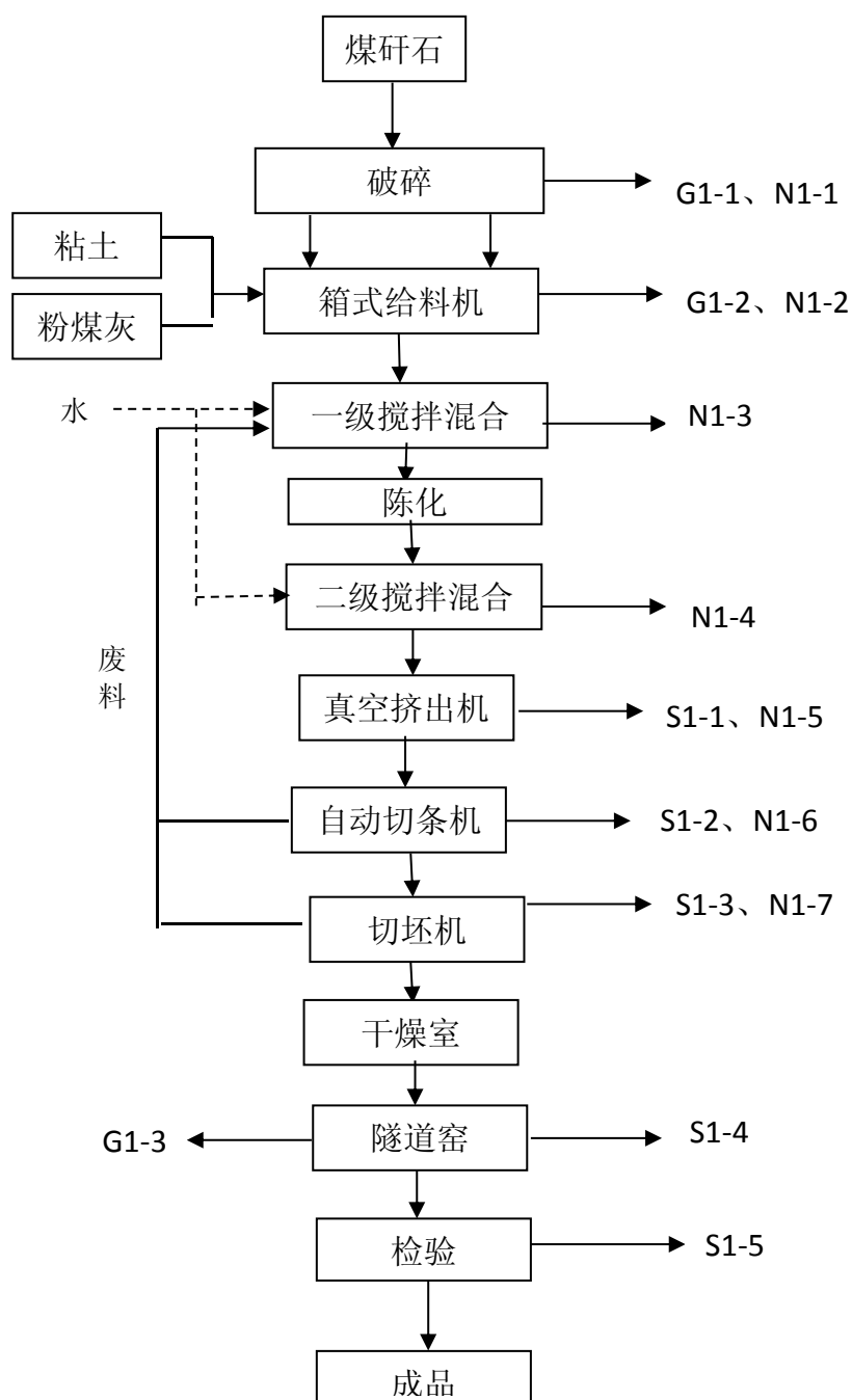
图3-3 项目工艺流程及产污环节图
