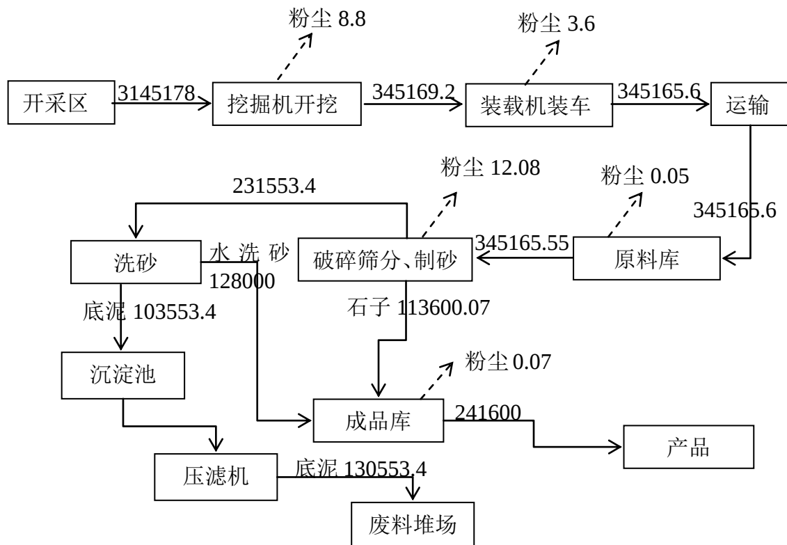
图 2.2-3 项目物料平衡图 单位: t/a
