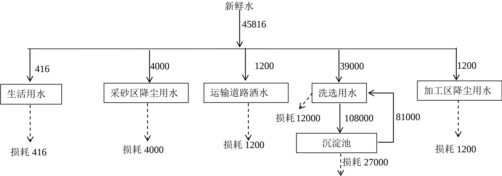
图 2.1-4 项目水平衡 单位：m³/a
